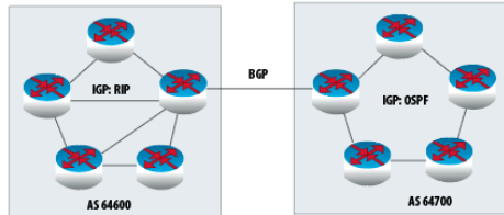
Figura 1.1. Protocolos de enrutamiento al interior y entre sistemas autónomos
