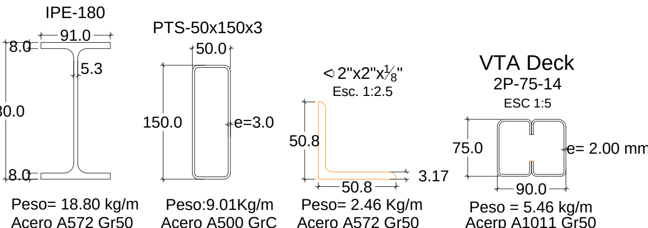
SECCIONES METÁLICAS Medidas en mm ESC 1:5
