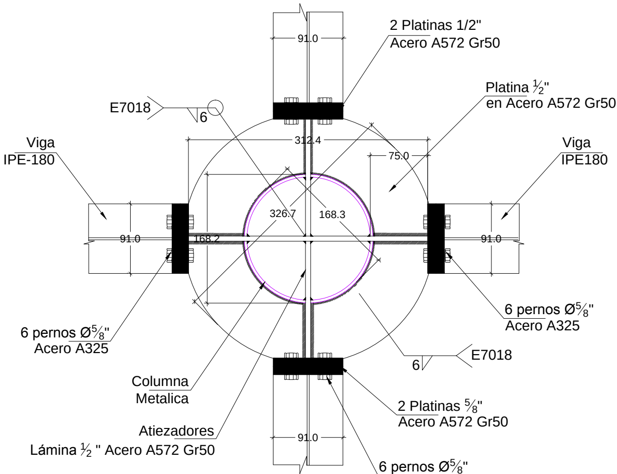
CONEXIÓN TIPO 2 ESC. 1:5 medidas en mm CORTE 1-1
