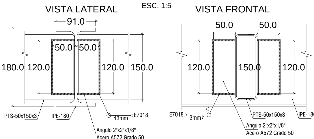
CONEXION 1 PTS a IPE medidas en mm ESC. 1:5
