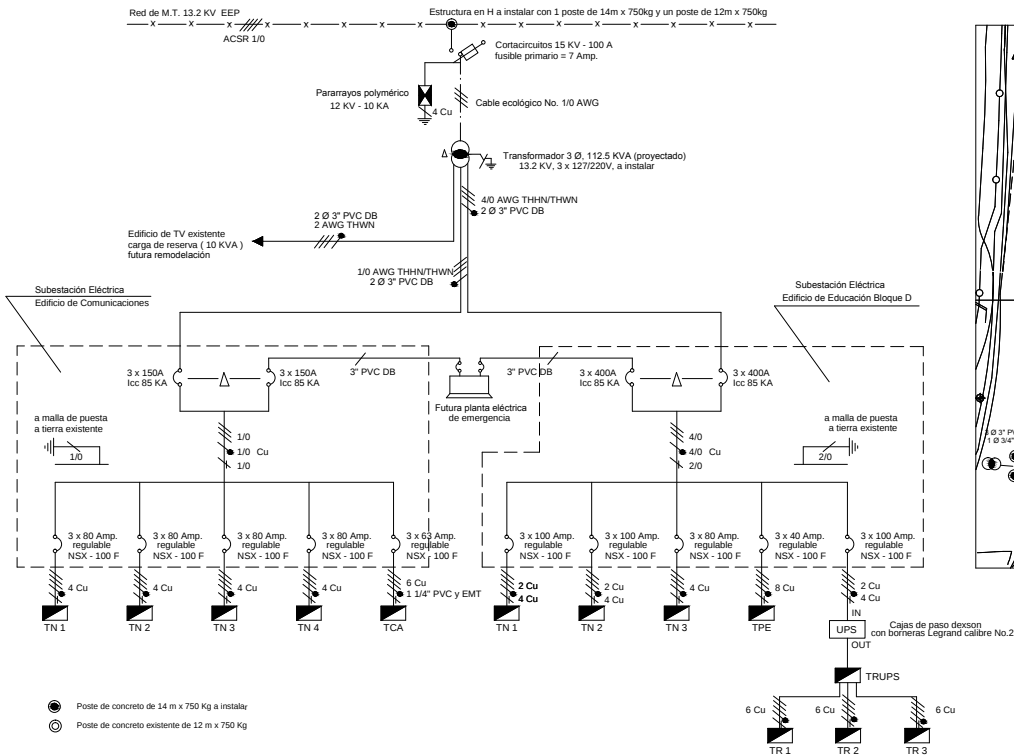
Diagrama Unifilar General Edificio de Comunicaciones y Edificio de Educación Bloque D
