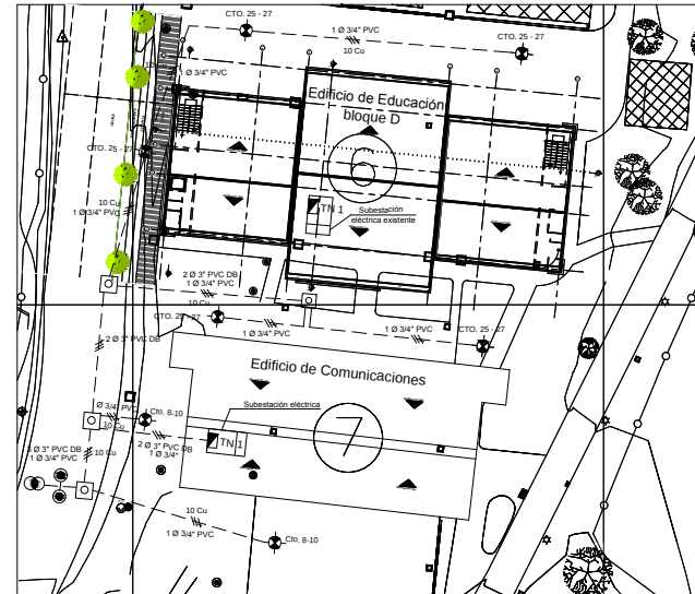
Localización Alumbrado Exterior
