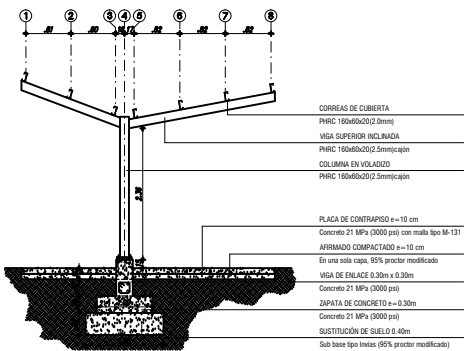
ALZADO GENERAL
