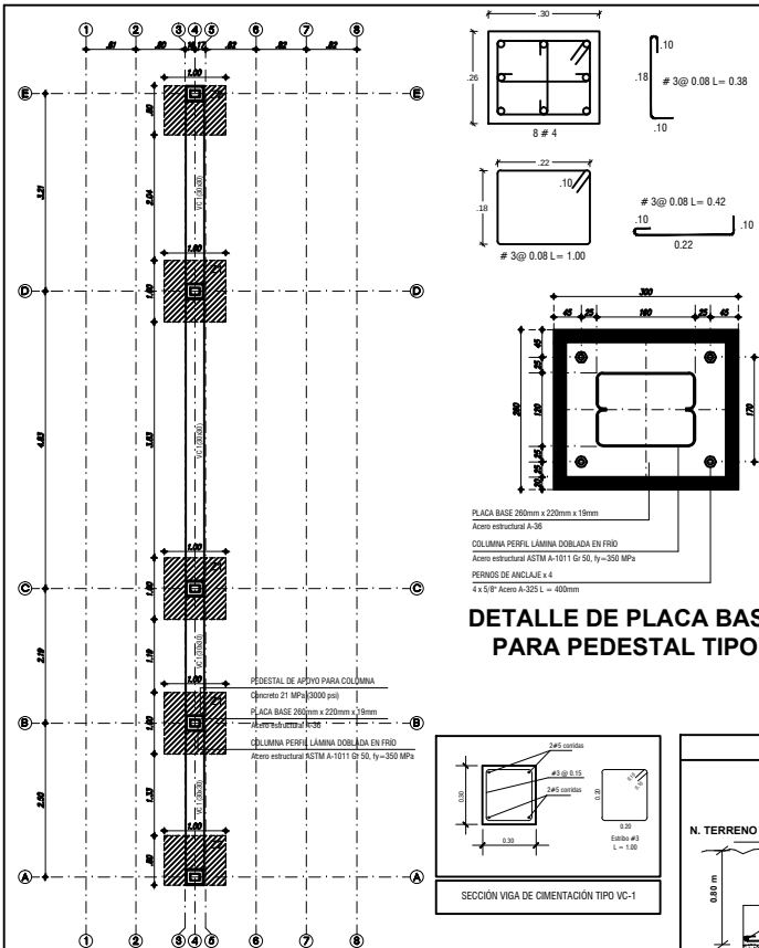
PLANTA DE CIMENTACIÓN
