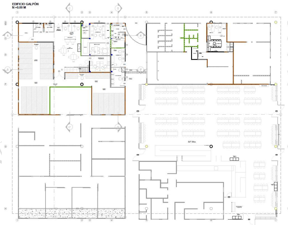
Plano Arquitectónico Galpón N+0.00 M
