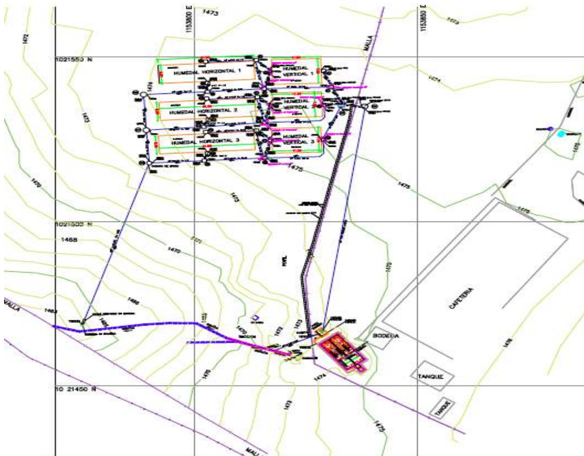
PLANTA TOPOGRÁFICA PLANTA DE TRATAMIENTO DE AGUAS RESIDUALES "PTAR" BELLAS ARTES
