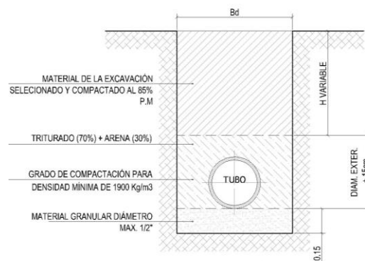
CIMENTACIÓN PARA TUBERÍA DE P.V.C
