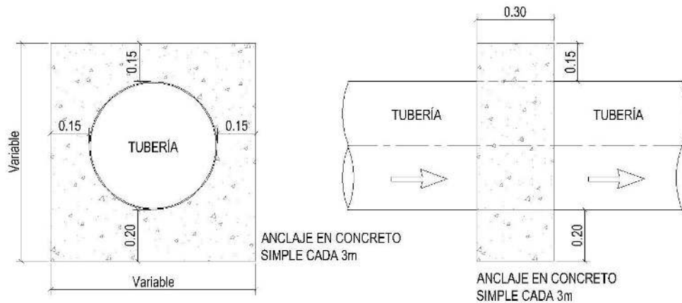
DETALLE ANCLAJE DE TUBERÍA P.V.C CON PENDIENTES MAYORES A 15%
