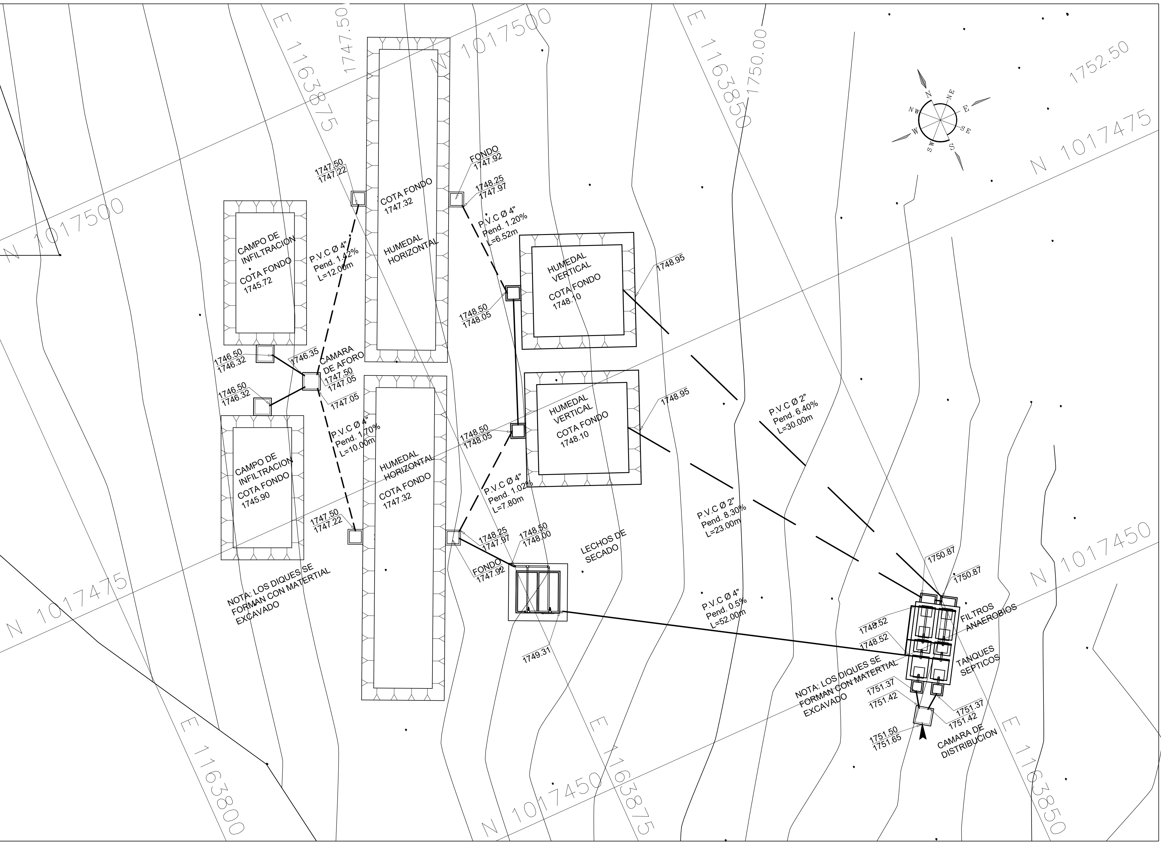
LOCALIZACION DETALLADA ESCALA 1:250
