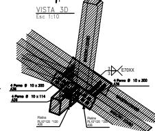
VISTA 3D Esc 1:10
