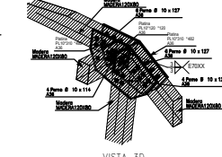
VISTA 3D Esc 1:10
