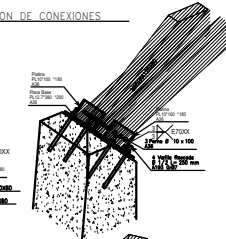
VISTA 3D Esc 1:10
