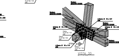
DETALLE CONEXIÓN 5 Esc. 1:10
