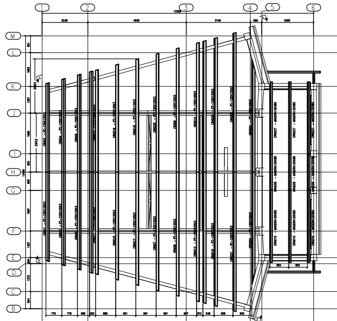
PLANTA CORREAS DE CUBIERTA N+5800 Esc: 1:50
