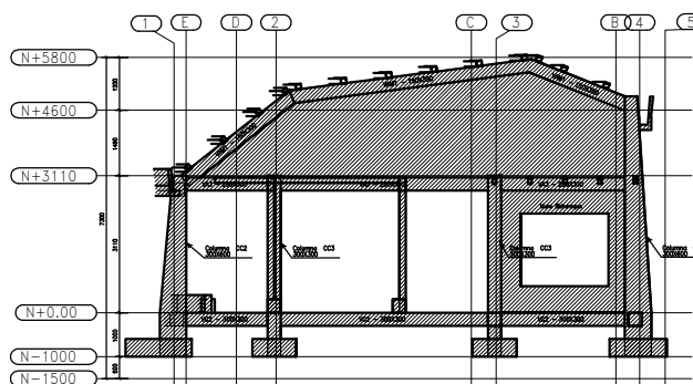
CORTE B-B En 1:50
