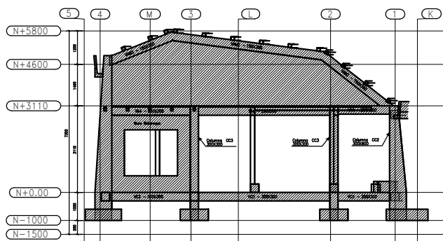
CORTE A-A En 1:50
