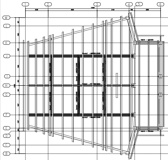
PLANTA VIGAS DE CUBIERTA N+5800 Esc: 1:50
