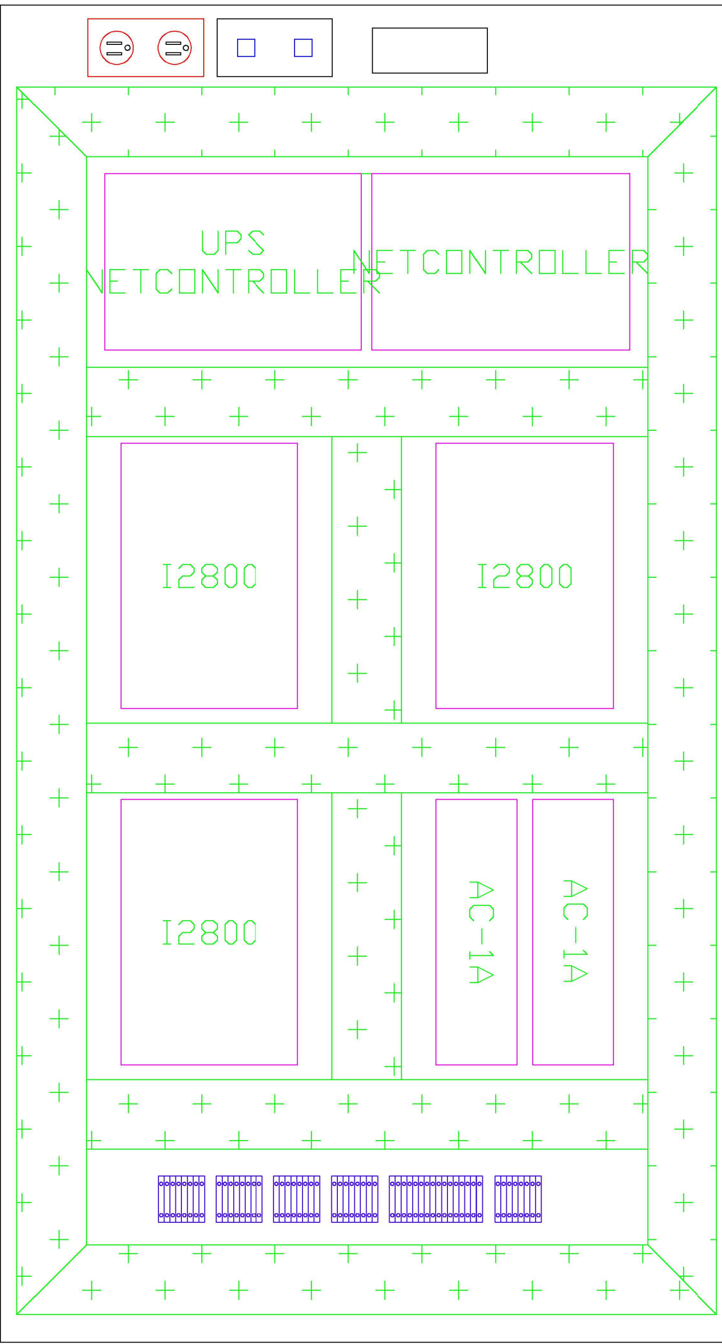
Distribución tablero principal de control
