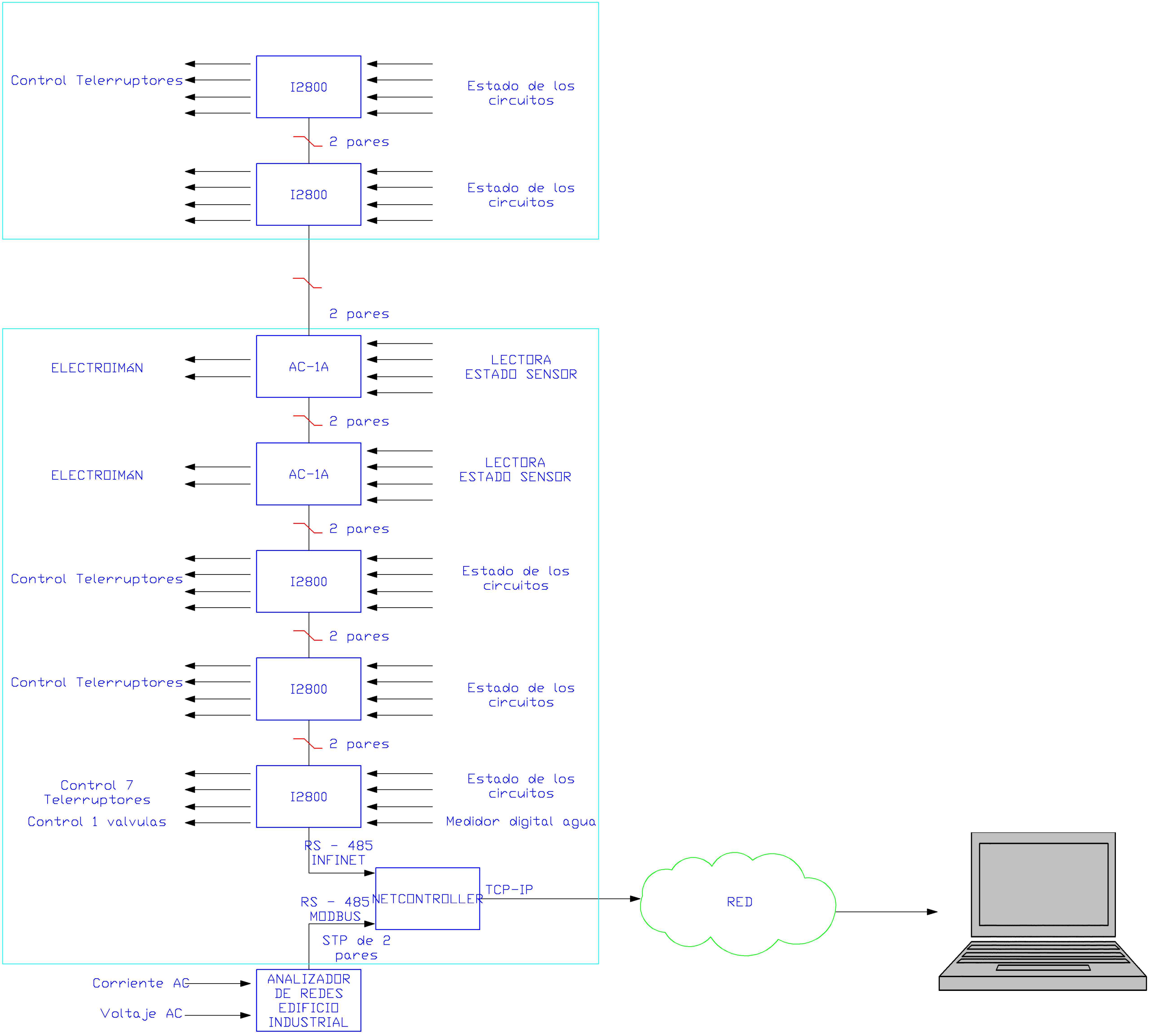
Diagrama de Interconexión
