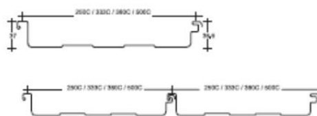
PERFIL DE LAS TEJAS
