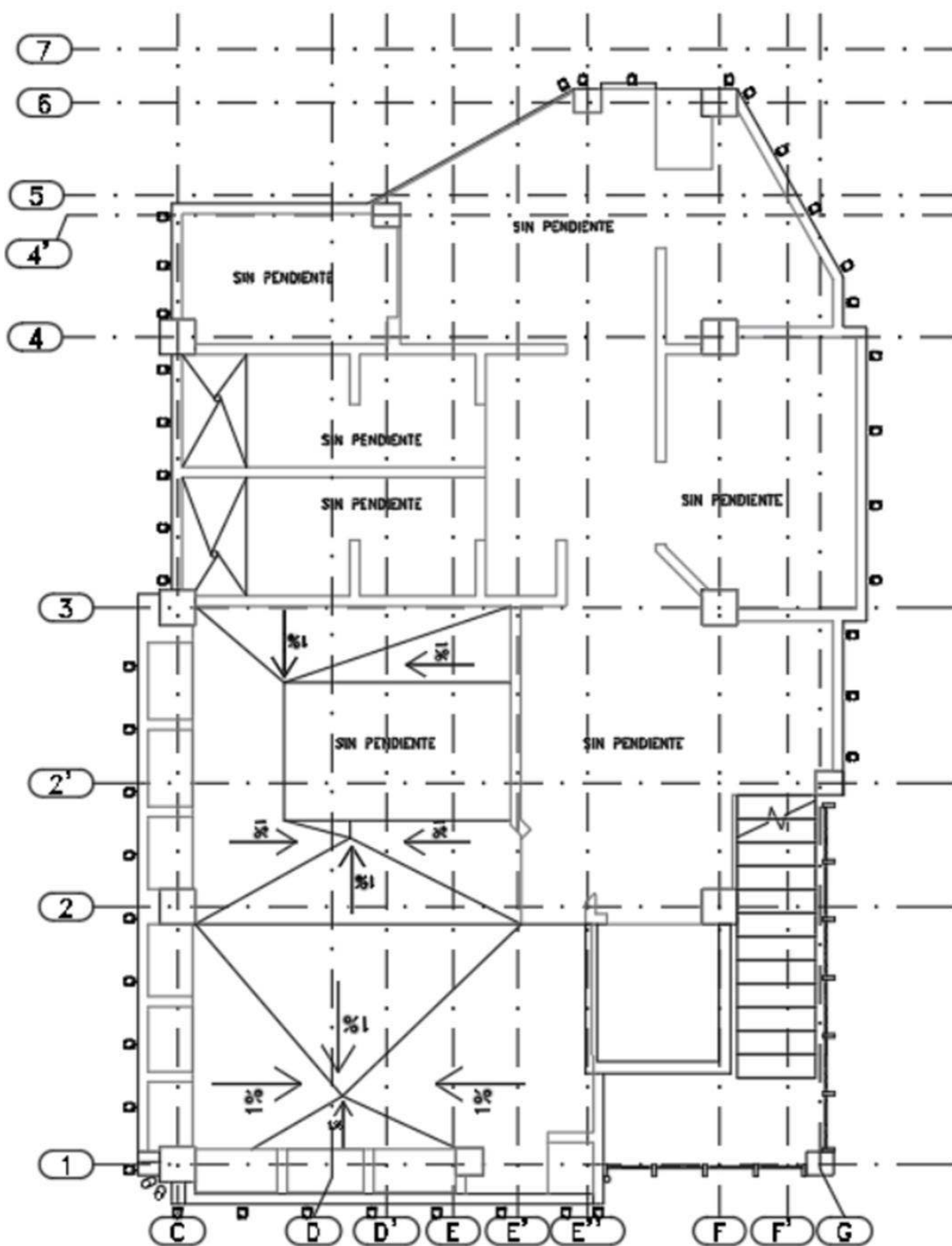
NIVEL 3.50 DESNIVELES PLACA ENTREPISO
