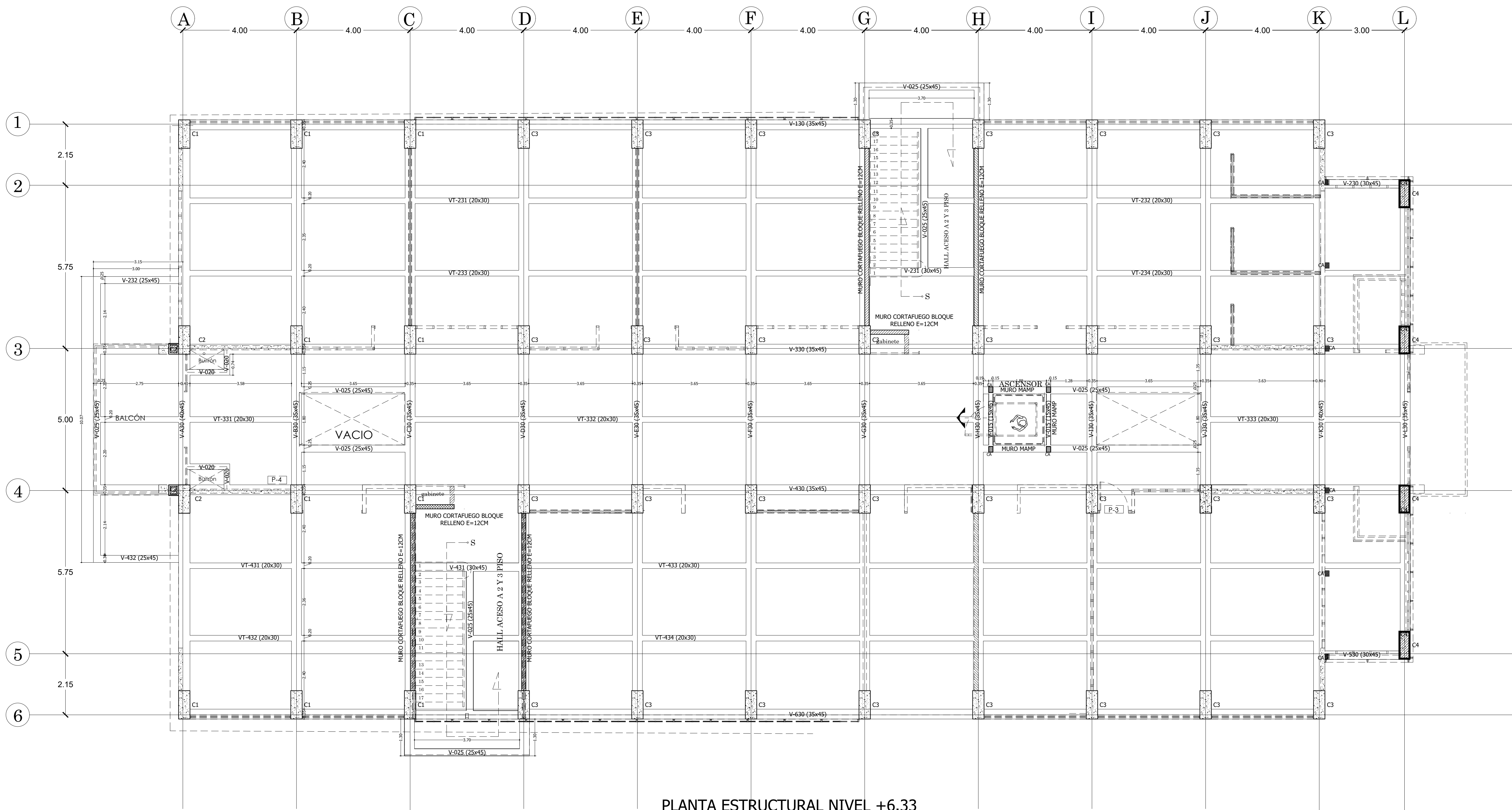
PLANTA ESTRUCTURAL NIVEL +6.33
