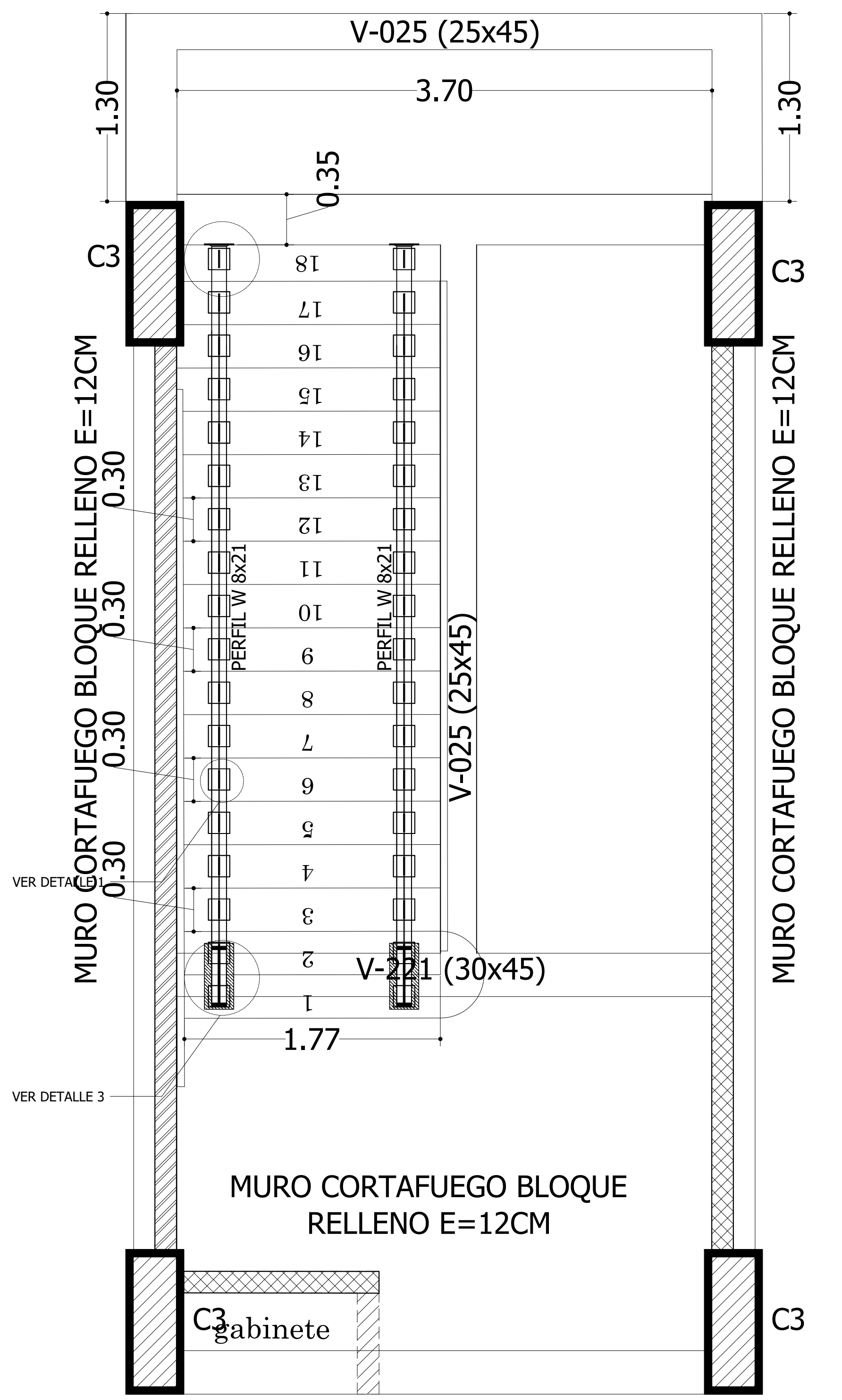
VISTA EN PLANTA ESCALERA METALICA NIVEL +0.03, +3.18 Y +6.33
