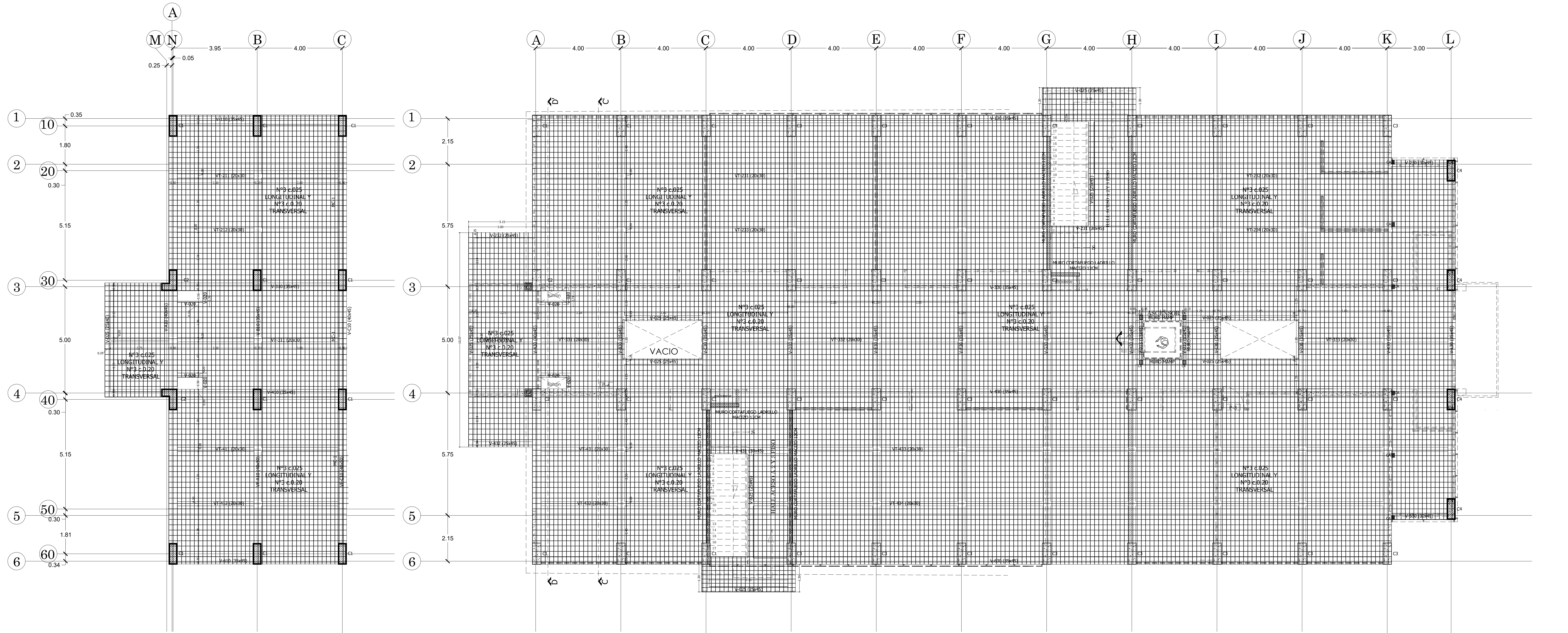
PLANTA REFUERZO INFERIOR LOSA N+0.03
