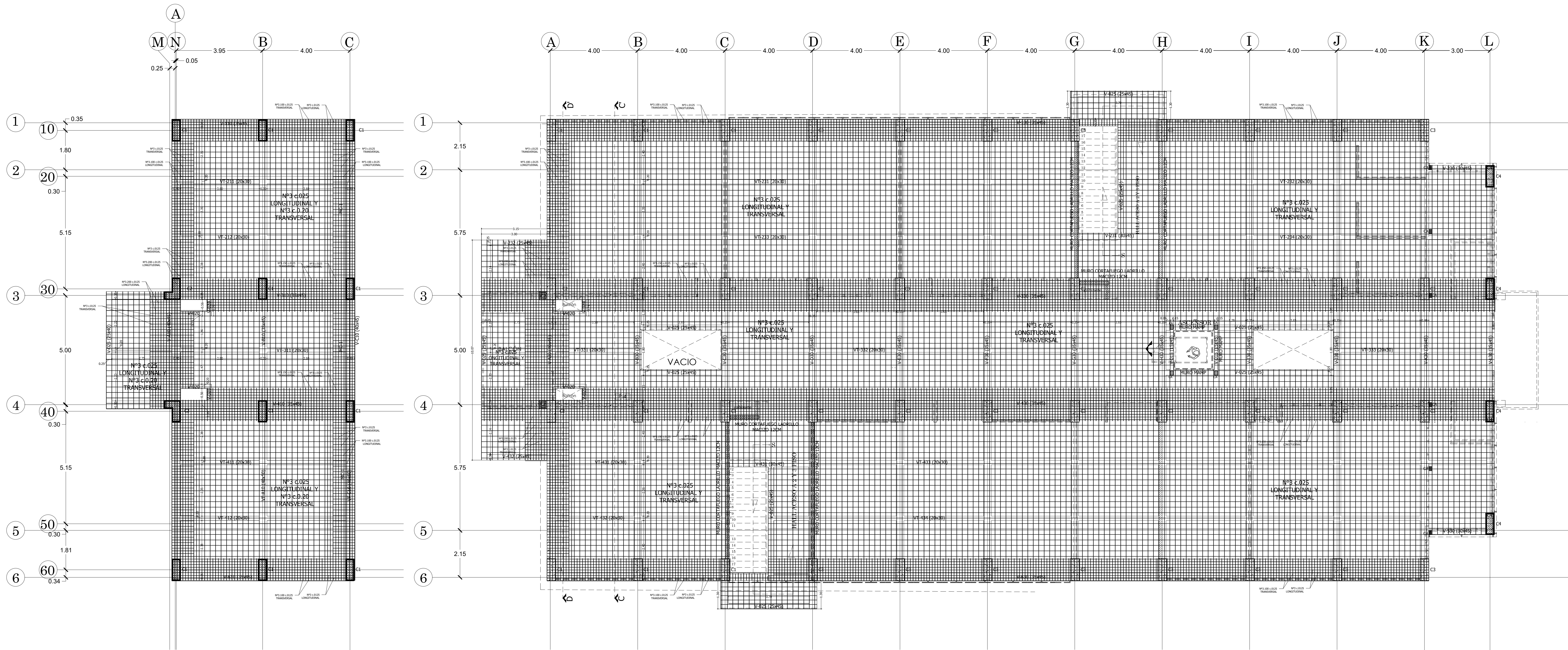
PLANTA REFUERZO SUPERIOR LOSA N+0.03
