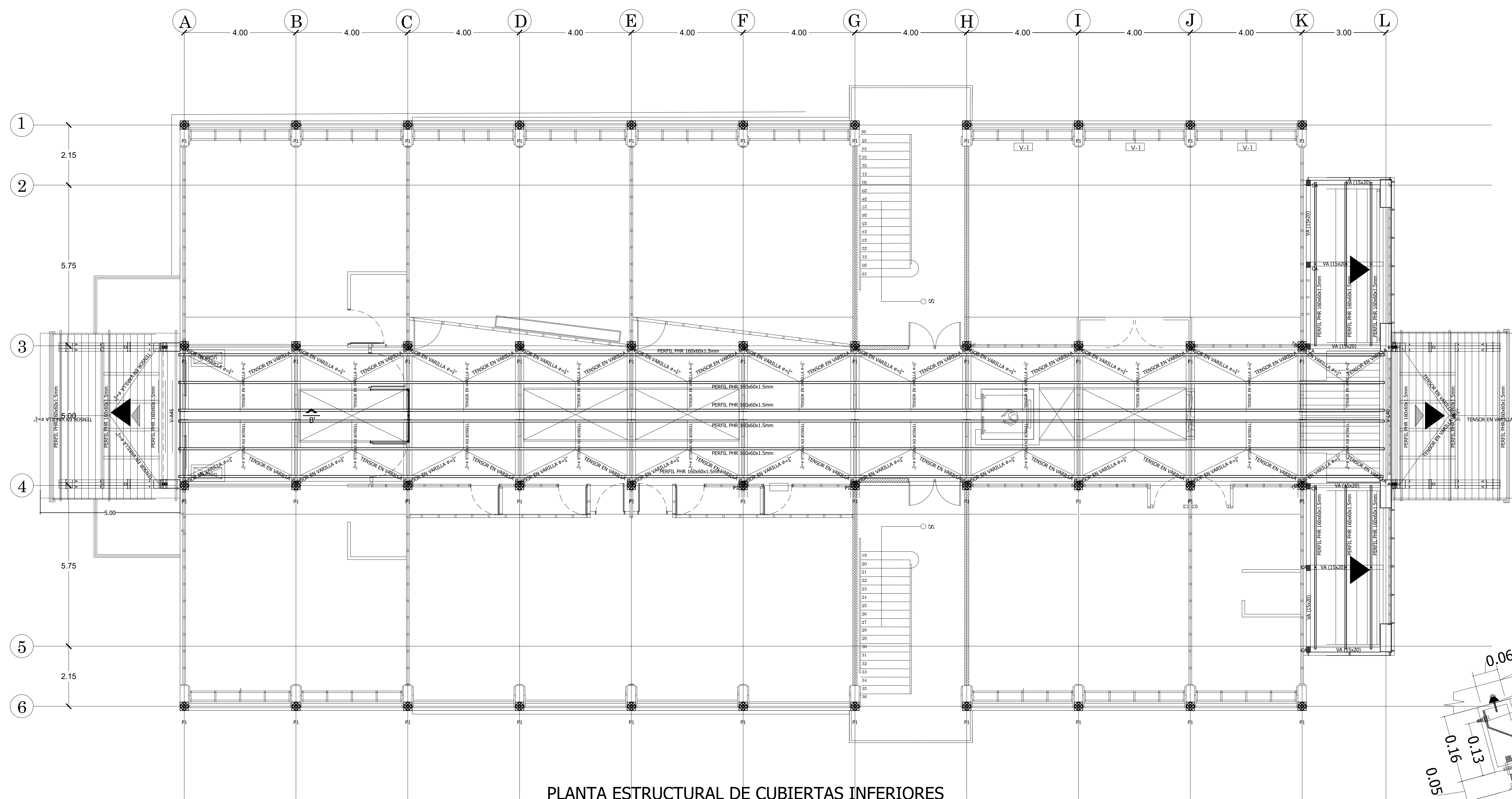
PLANTA ESTRUCTURAL DE CUBIERTAS INFERIORES
