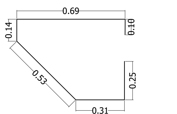
DESPIECES DE ESTRIBO DE MENSULA ESCALA 1:15
