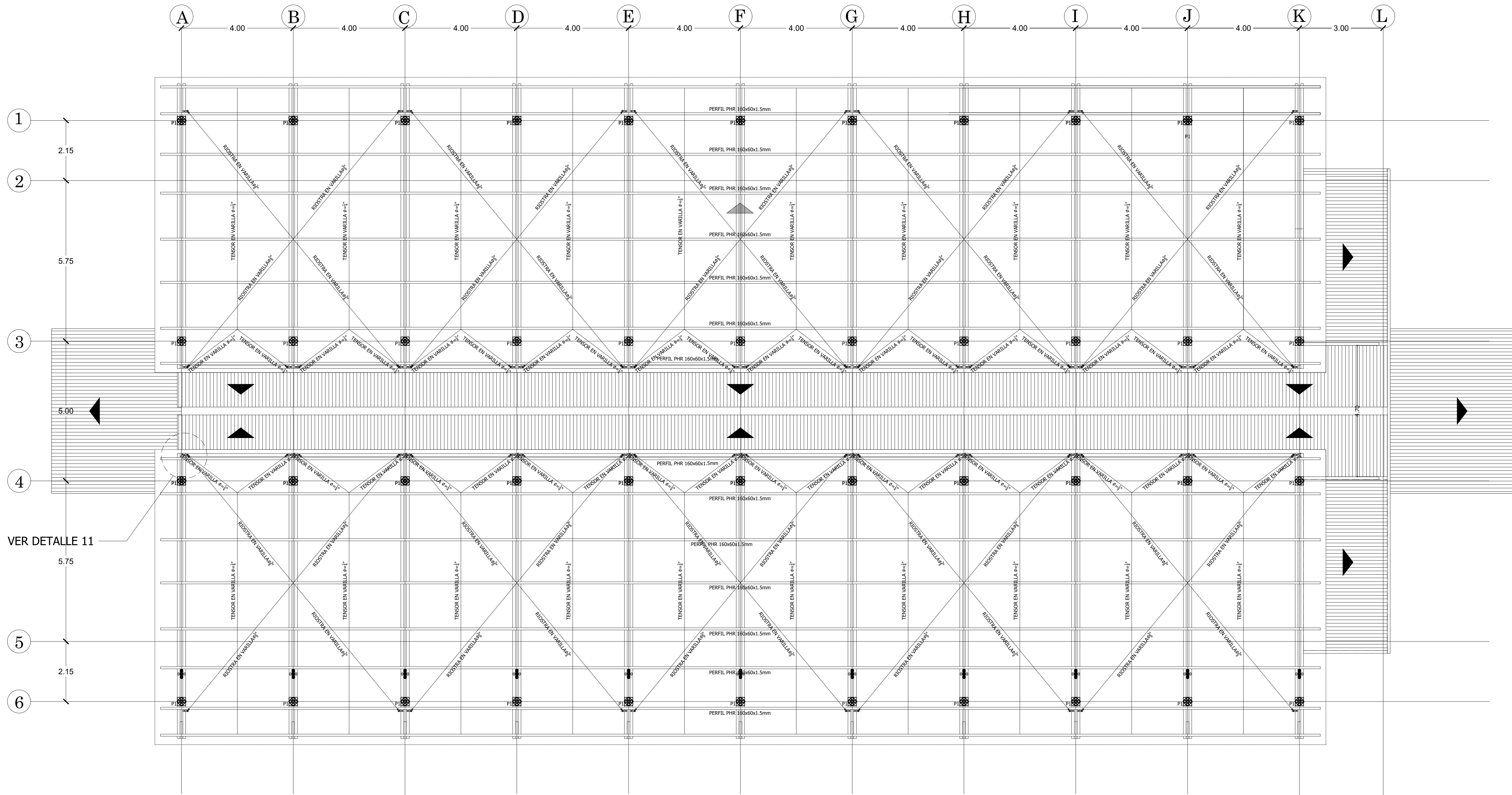
PLANTA ESTRUCTURAL DE CUBIERTAS SUPERIORES
