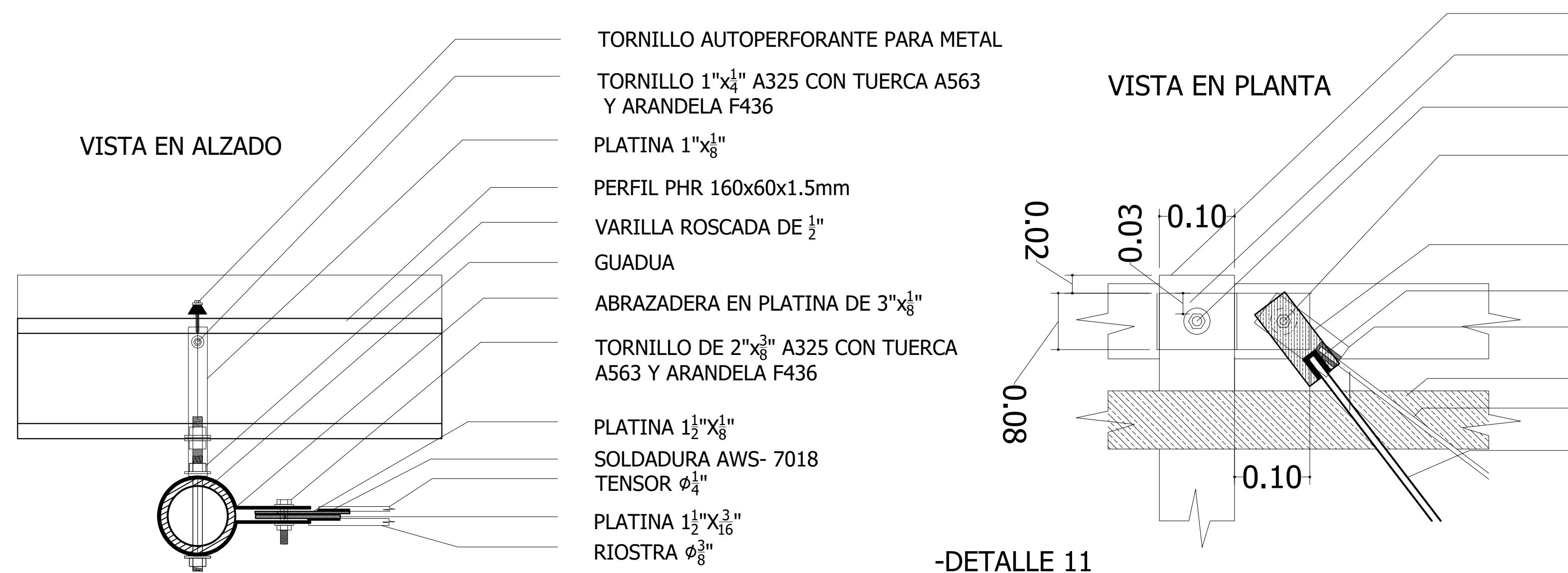
-DETALLE 11 ANCLAJE TENSORES Y RIOSTRAS DE CUBIERTA ESCALA 1:5
