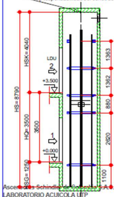
Sección Vertical 1:100
