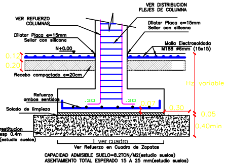
DETALLE CIMENTACION
