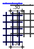
DETALLE TRASLAPO DE MALLA ELECTROSOLDADA
