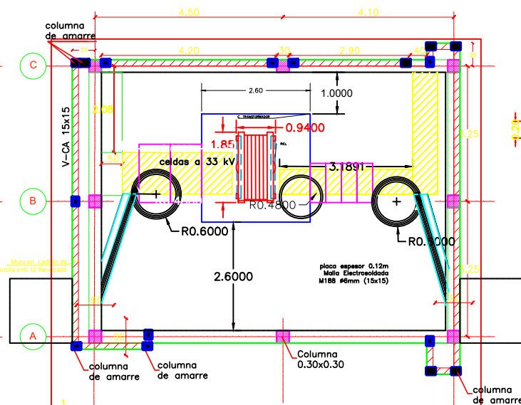
PLANTA PLACA CONTRAPISO
