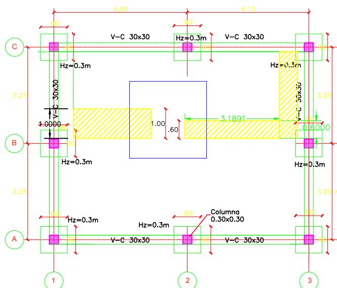
PLANTA CIMENTACION
