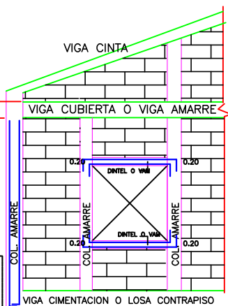
DETALLE MUROS NO ESTRUCTURALES Y CULATAS APOYO CUBIERTA EJES 1 Y 3
